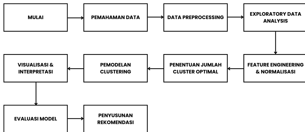
Gambar 3.1.1 Alur Kerja
