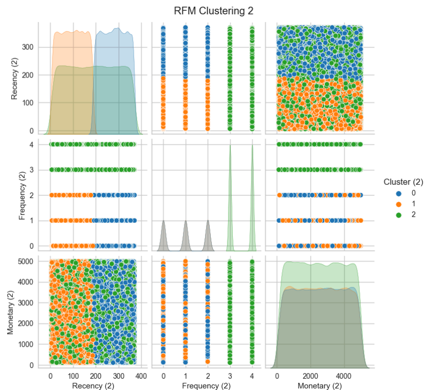
Gambar 4.3.2 Cluster Kombinasi 2
