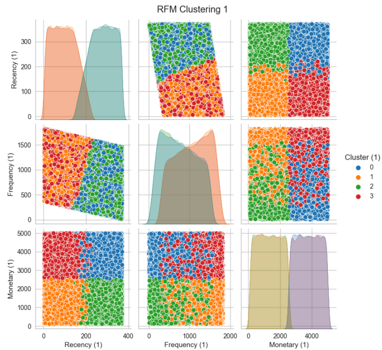
Gambar 4.3.1 Cluster Kombinasi 1
